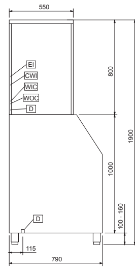
Zij aanzicht
