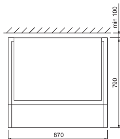
Boven aanzicht
